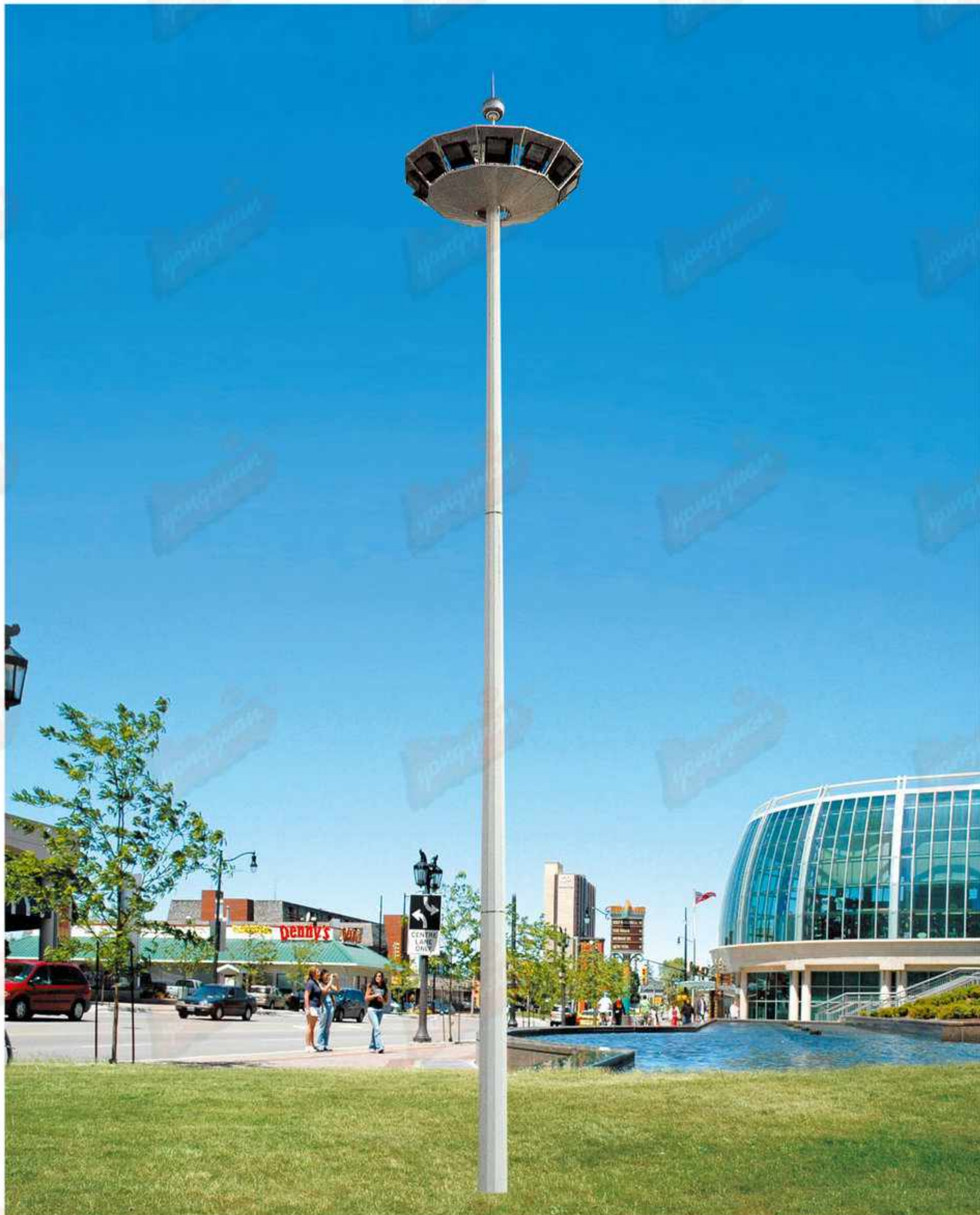
型号：永安名牌2019A25 技术参数：总高18-30m，钢铁制品；灯具铝制品，配400w-1000w高压钠灯，金卤灯或LED光源，全套内外热浸锌防腐处理后喷优质户外氟碳漆，配置高杆灯专用自动升降系统，配钢丝绳、电缆线、地基螺丝及提供安装技术指导，具体技术规范根据安装地域的抗风等级及地震烈度设防度的要求。
