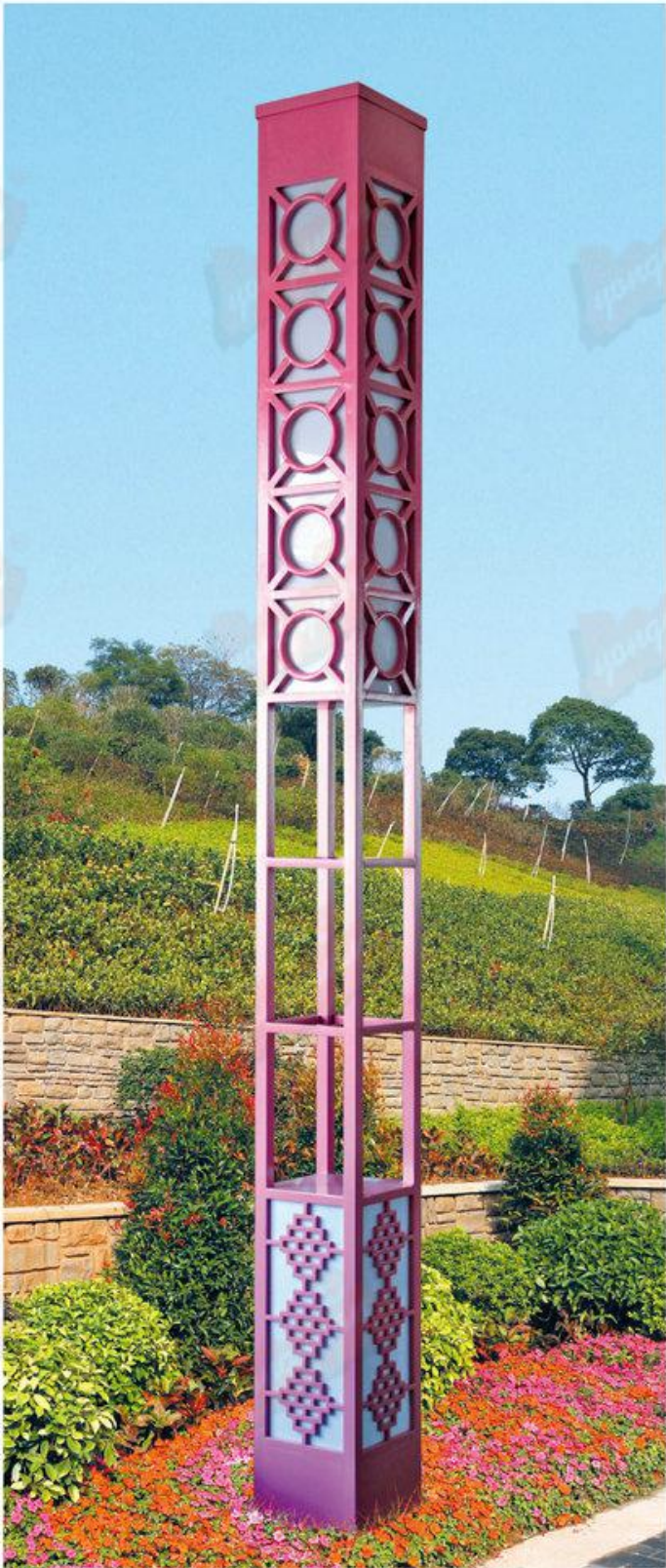
型号：永安名牌2019F77 技术参数：总高3-6m，钢铁、不锈钢制品；配LED光源或节能光管，灯体喷优质户外氟碳漆或户外塑。
