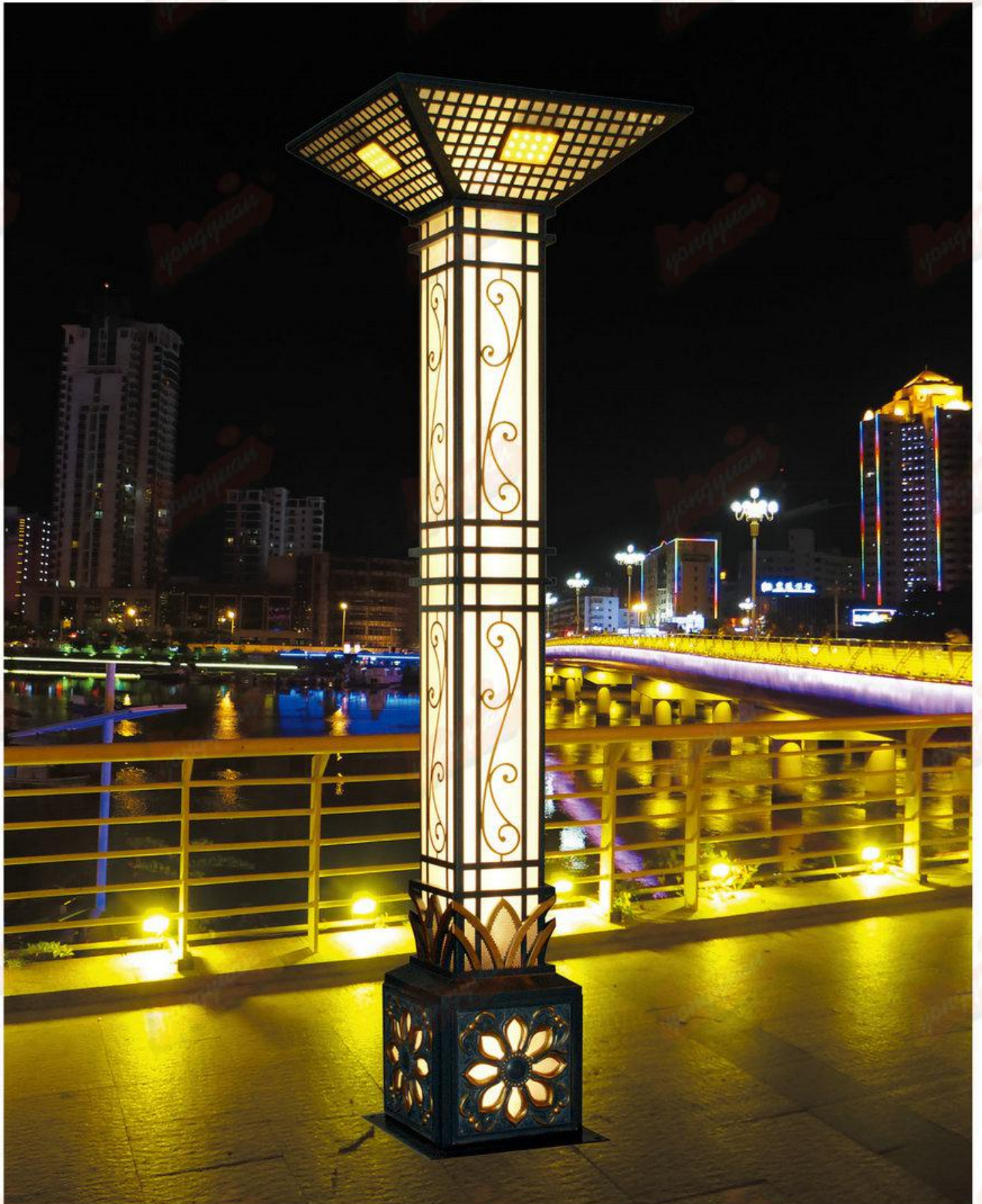
型号：永安名牌2019F27 技术参数：总高3-6m，不锈钢201或304材质，装饰花为沙铸铝制品，灯体喷优质户外氟碳漆，配LED光源或节能光管。
