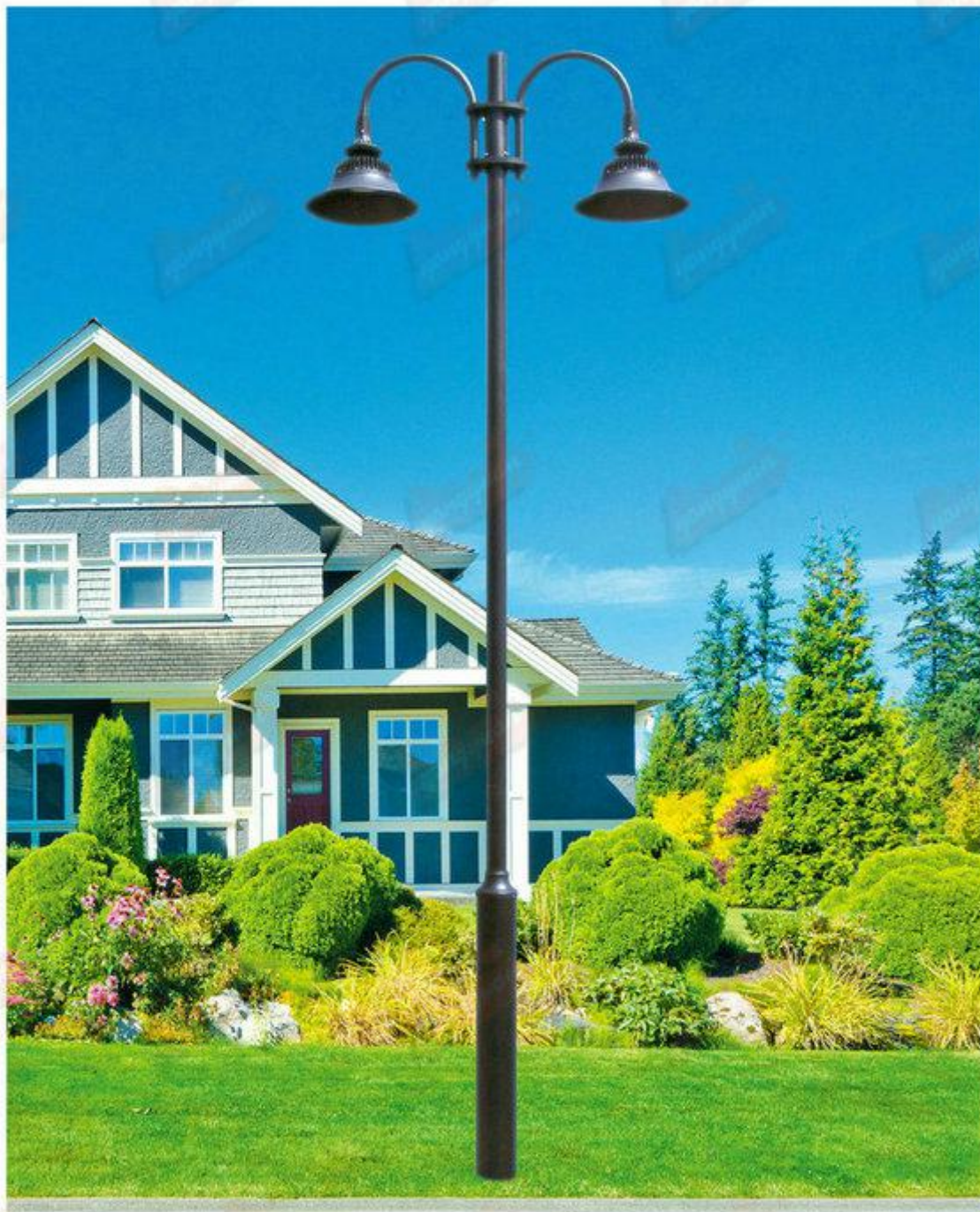
型号：永安名牌2019H508 技术参数：总高3-6m，钢铁制品；灯具铝制品，配LED灯光源，灯体内外热浸锌防腐处理后喷优质户外氟碳漆。
