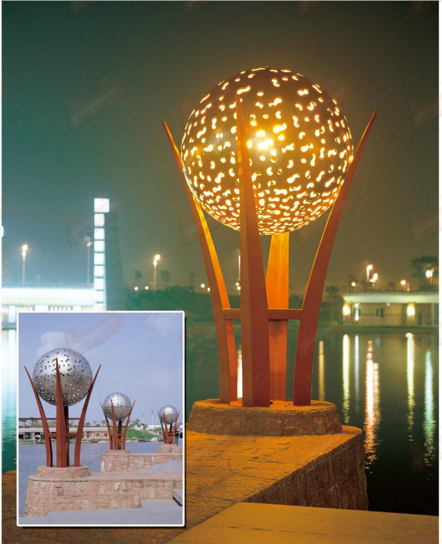
型号：永安名牌2019F323 技术参数：总高1.5-3m，钢铁、不锈钢制品；配70W、150W、250W、400W钠灯，灯体内外热浸锌防腐处理后喷优质户外氟碳漆，灯体材料为Q235、SS400可供选择。
