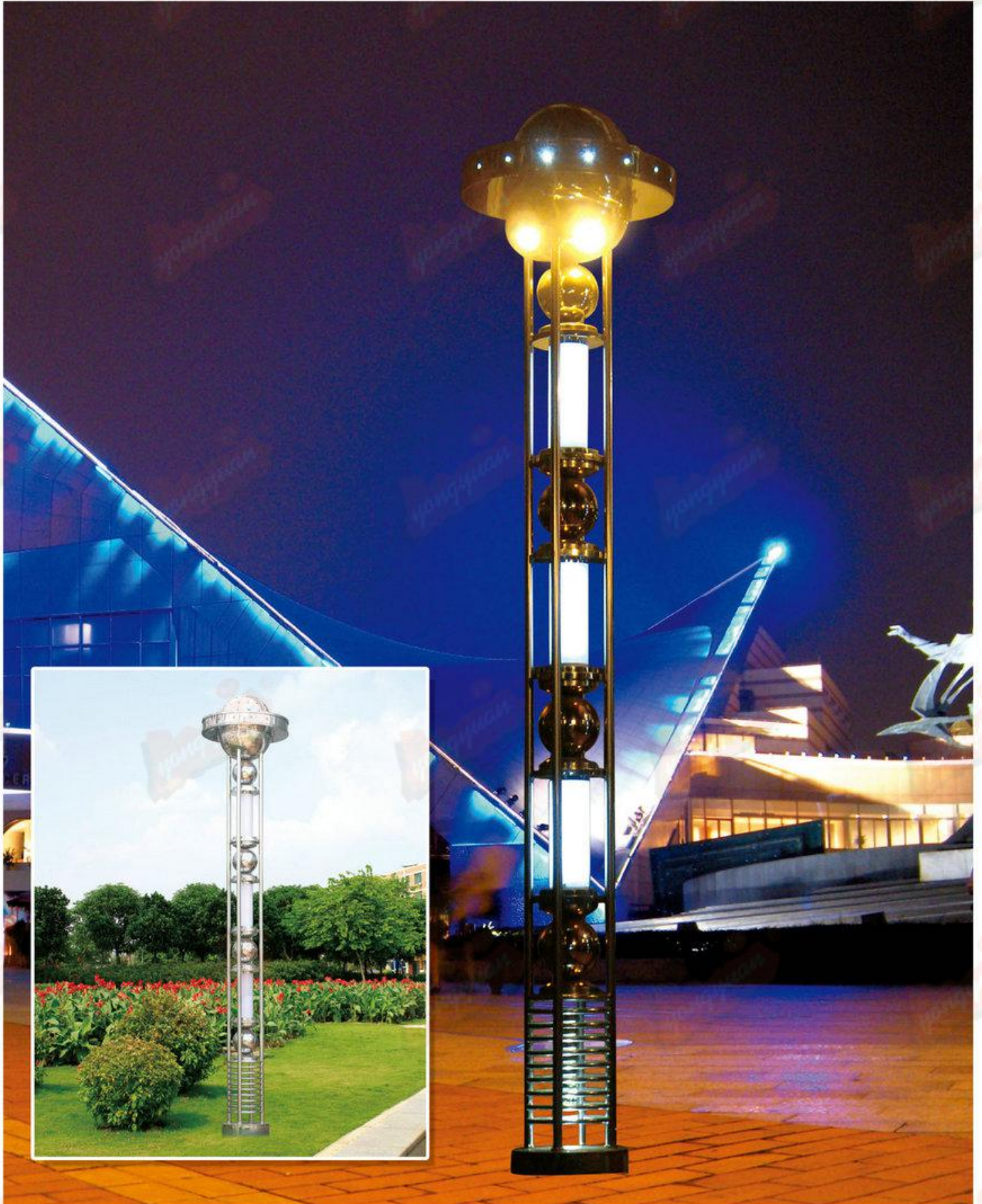
型号：永安名牌2019F349 技术参数：总高6-8m，不锈钢制品；配LED光源或节能光源，不锈钢材质分为200系列、304系列。
