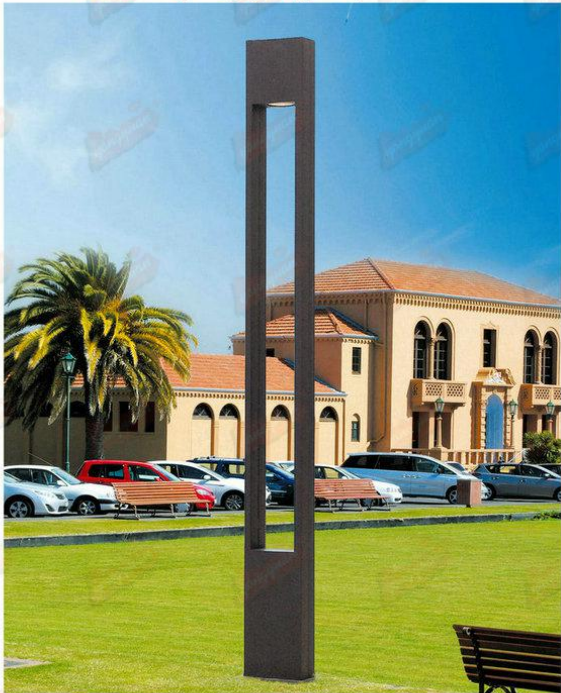
型号：永安名牌2019H281 技术参数：总高3-5m，铁铝制品；灯体内外热浸锌防腐处理后喷优质户外氟碳或户外型。
