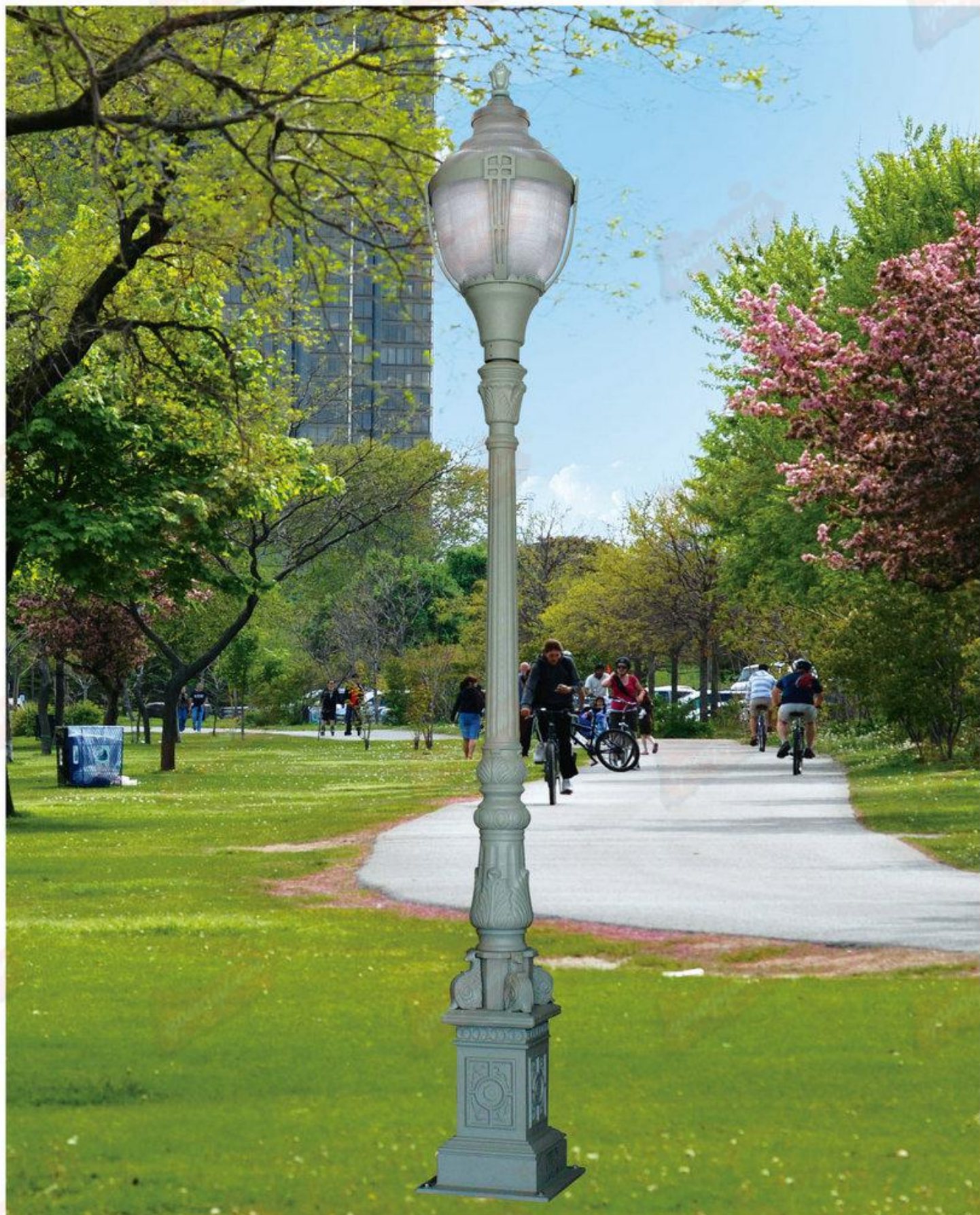
型号：永安名牌2019G1032 技术参数：全套铝制品。总高：小号模具有：3米、3.3米、3.5米。中号模具有：3.8米。大号模具有：4.3米、4.8米、5.3米。 配PMMA灯罩，配全套喷永安优质户外塑或户外氟碳漆。
